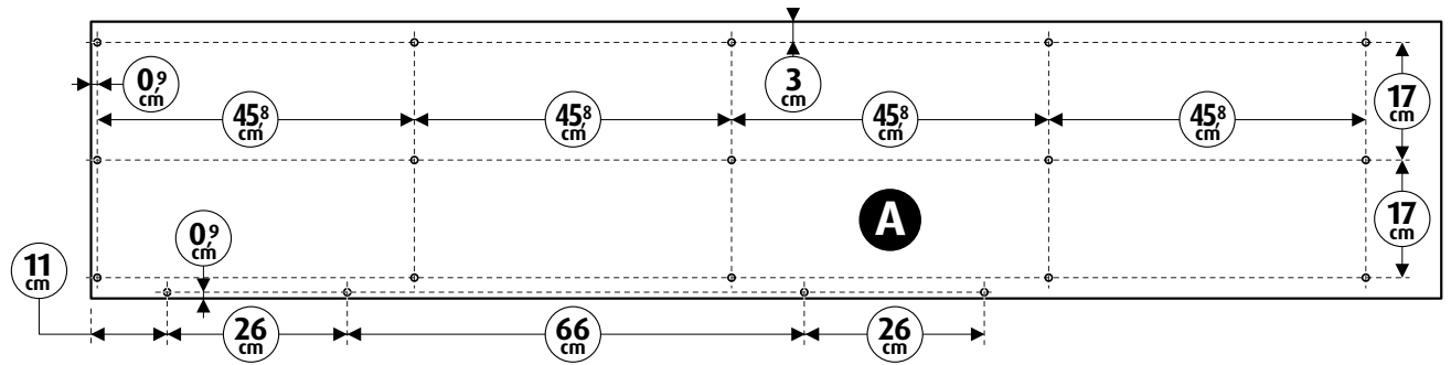
Boorplan zitting 40 x 195 cm Gaten voorboren \varnothing 4 mm en verzinken
